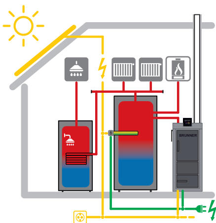
BRUNNER Scheitholzheizung mit separaten Warm- und Heizwasserspeicher. Die Systemsteuerung regelt alle Kessel und Heizfunktionen. Solarstrom lässt sich über die BRUNNER Fotovoltaikbindung zum Heizen nutzen (Elektrostab).
